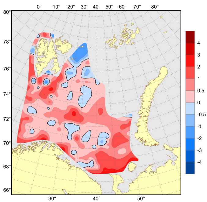
Figure 4.1.1.10. Bottom temperature anomalies (°C), August–November 2022.
