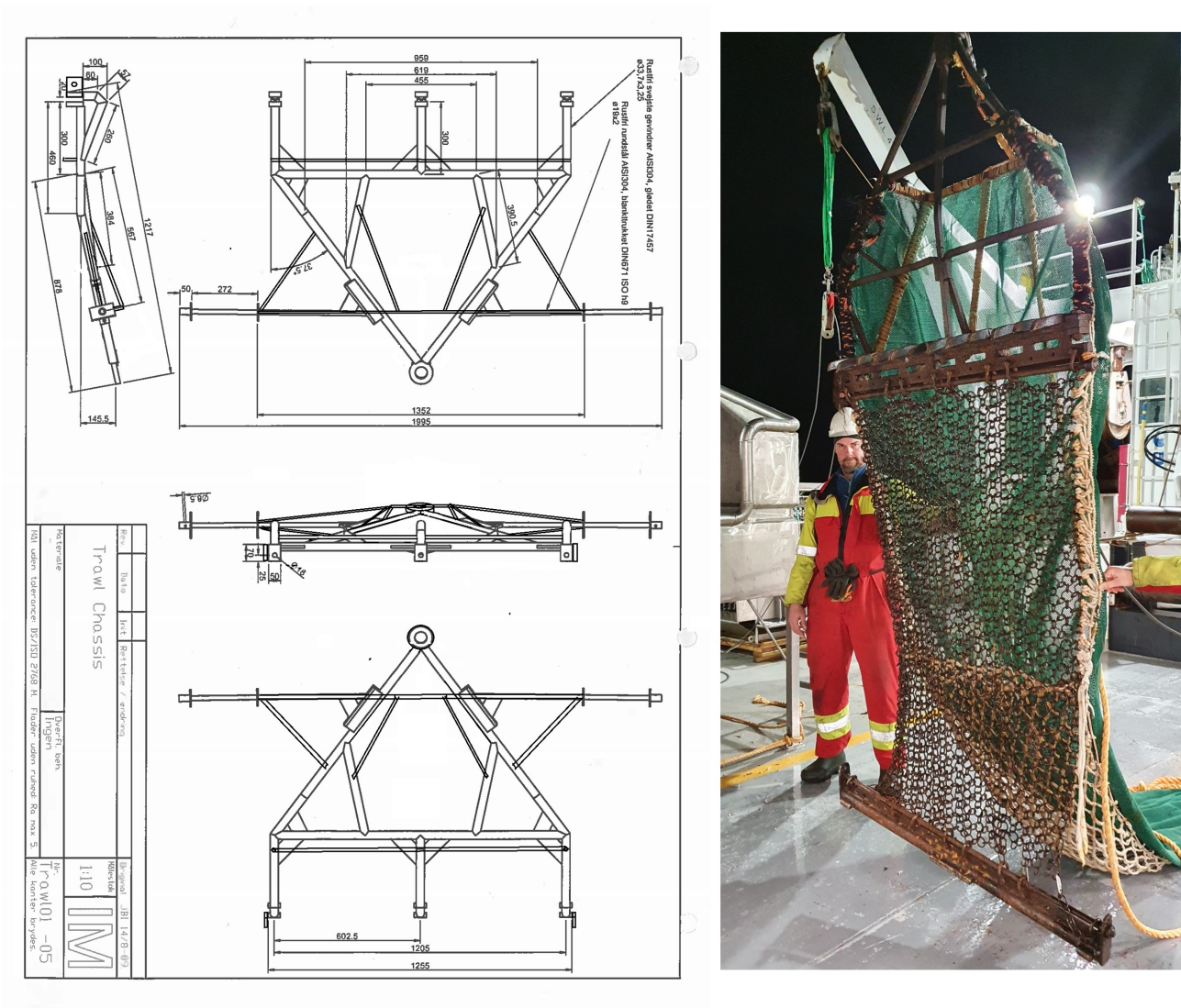
Vedleggsfigur 1. Skisse og foto av tobisskrapen som ble benyttet under toktet.
