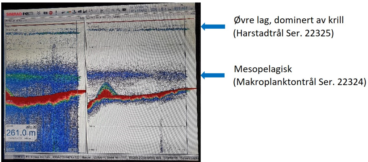
Figur 6.52. Akustisk registrering ved krillstasjon i Høyangsfjorden, 15.02.2022 (nattstasjon).
