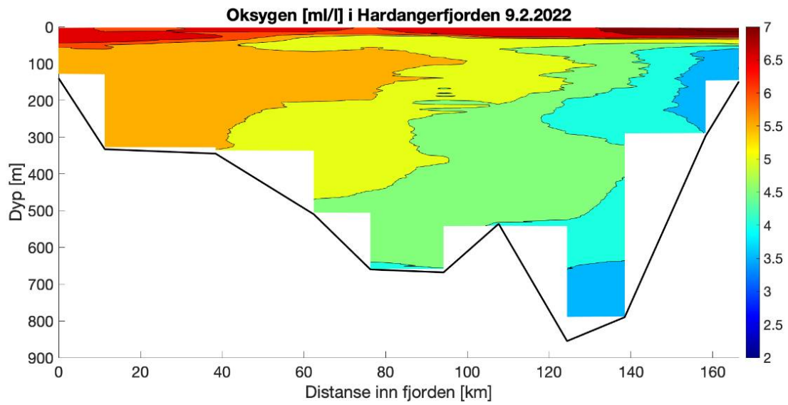
Figur 6.6. Oksygenivå innover i Hardangerfjorden.
