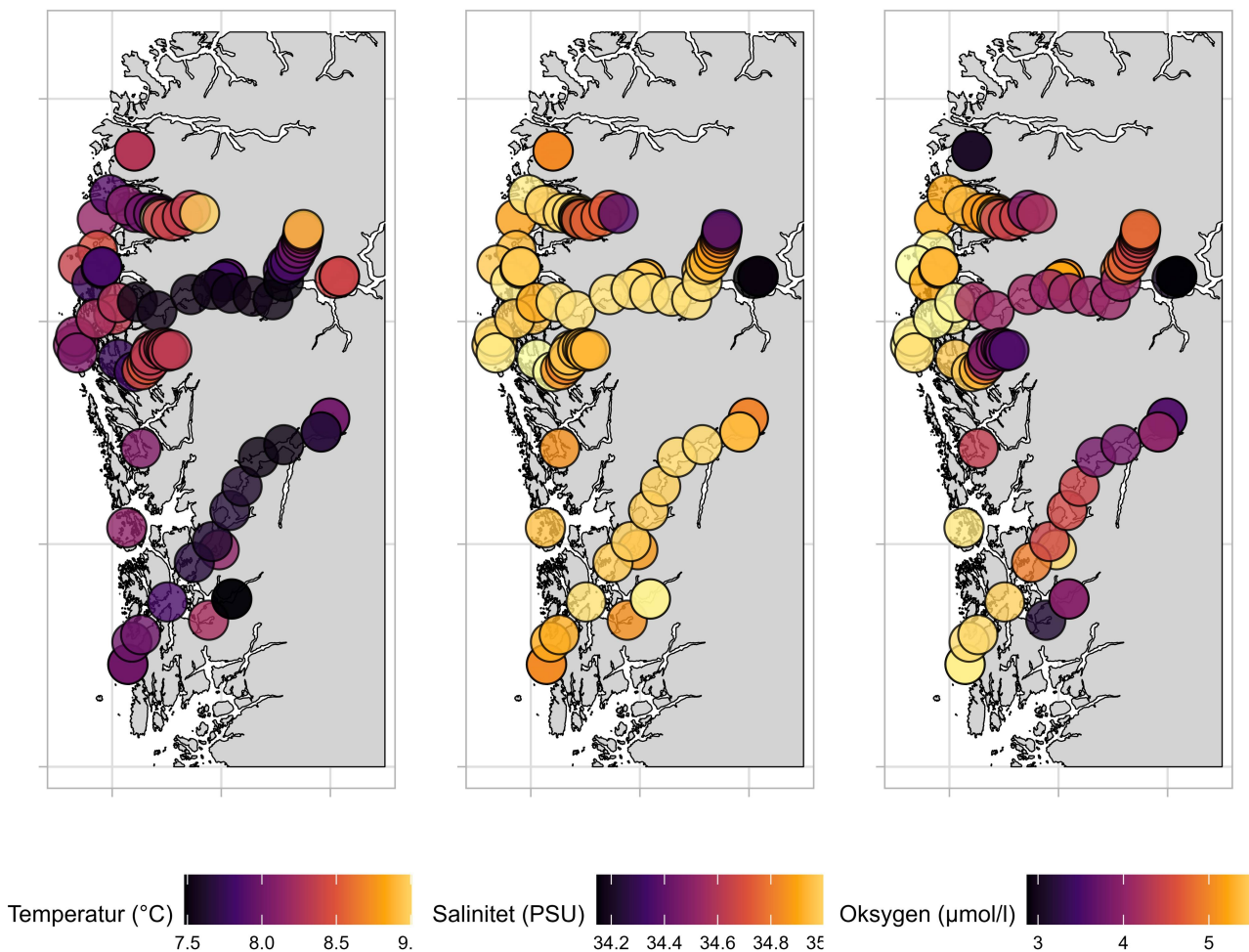
Figur 6.3. Temperatur, salinitet og oksygeninnhold i bunnvannet på alle CTD-stasjonene.
