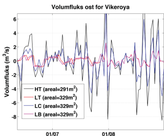
Figur 24. Tilsvarende som for Figur , men tidsseriene her representerer volumfluks gjennom et transektet hvor det er smalest mellom Vikerøya og fastlandet på sørsiden av øya.
