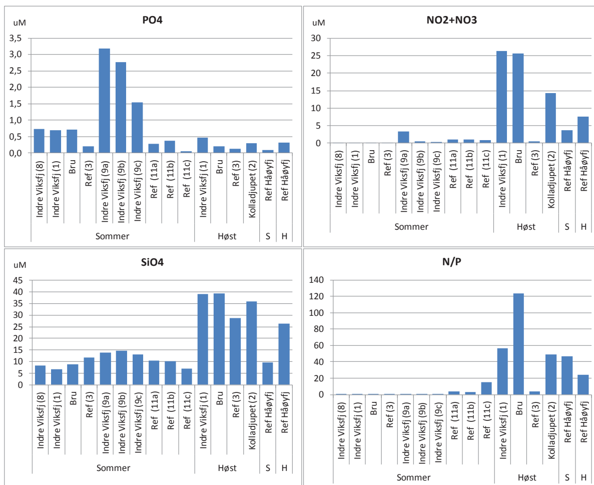
Figur 14. Næringssalter (fosfat (PO 4 ), nitrat (NO 2 +NO 3 ) og silikat (SiO 4 )) i vannprøver fra Indre Viksfjord og referanseområder utenfor, jfr kart i Figur 13, samt forholdstallet mellom fosfat og nitrat.
