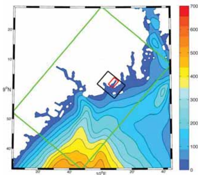
Figur 19. Bathymetriske kart over Vestfold og omegn som viser utstrekningen til de høyoppløselige strømmodellene for Vestfold (200m oppløsning, grønn rute), Larvik (50m, svart rute) og Viksfjorden (10m, rød rute). Utstrekningen til den utenforliggende 800m-modellen er ikke vist, men denne omfatter hele Skagerrak inkludert Vestlandet.
