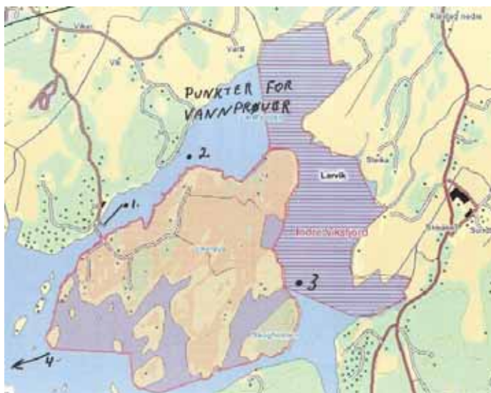
Figur 34. Vannprøvestasjoner i 2013. Stasjonsposisjoner:
