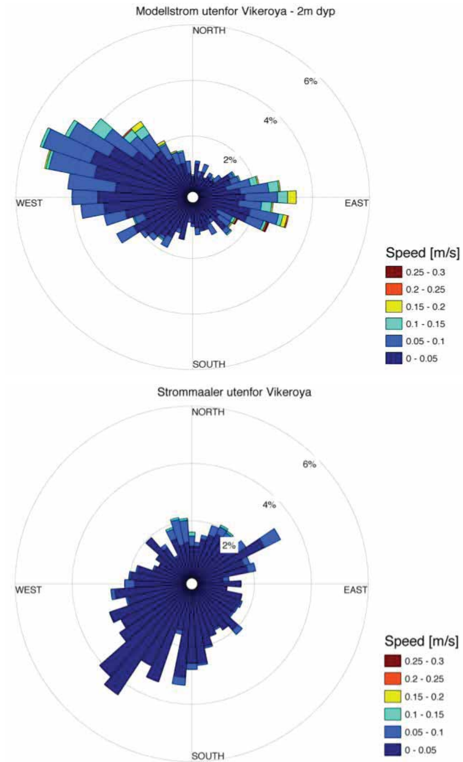
Figur 29. Strømrose fra målinger for perioden 23/10-23/11 2012 (øverst) og fra modell for perioden 10/6-31/8 2009 (nederst) fra posisjon angitt med nr. 8 på Figur 2 (utenfor Vikeroya). Strøm er målt/beregnet i ca. 2m dyp. Vinkelen i strømmrosene angir retning strømmen går mot, fargekodingen angir strømstyrken og lengden på sektorene angir hvor ofte retningen inntreffer.
