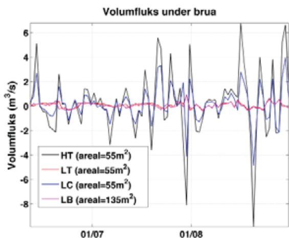
Figur 23. Tidsserie av volumfluks ( \text{m}^3/\text{s} ) gjennom simuleringsperioden fra 10/6 til 31/8 2009. Enkeltverdiene er beregnet ut fra døgnmidlet strøm midlet over alle dyp (tidevannsbevegelsen er derfor midlet bort). I tillegg er strømhastighet i hvert beregningspunkt multiplisert med arealet som denne representerer. Volumflukser er beregnet fra alle fire sensitivitetstester (angitt med farge) samt at arealet til hele transektet er angitt i forklaringen. Tidsseriene her representerer volumfluks forbi transektet hvor brua ligger.
