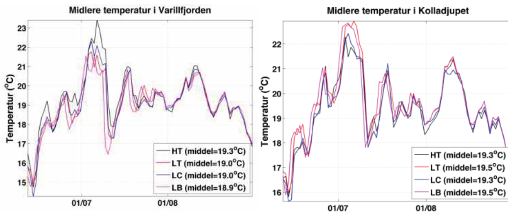
Figur 27. Modellert temperaturutvikling fra 10/6-31/8 2012 for et lite område i Varildfjorden (venstre side) og Kolladjupet (høyre side) midlet fra bunn til overflate. Kun døgnmidlete verdier er vist. Middelveidien for hele tidsserien er vist i forklaringen.
