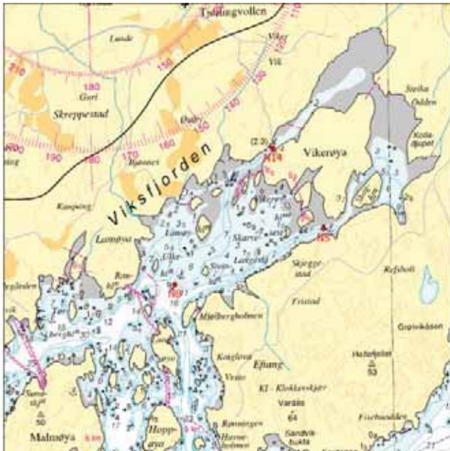
Figur 21. Bathymetriske kart fra Statens Kartverk Sjø over Viksfjorden og plasseringen av de tre strømmålerne.
