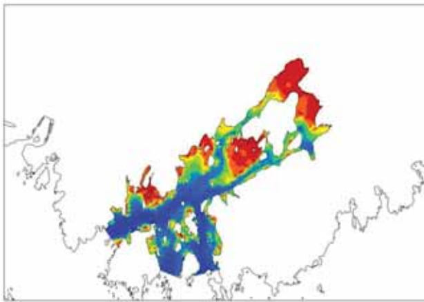
Figur 20. Bathymetriske modell (bunndyp) over Viksfjorden satt sammen av dybde data fra Norge Digitalt og multistråle-ekkolodd oppmåling utført av HI sommeren 2012. Rødtone indikerer arealer som tørrlegges på lavvann og blått vann dypere enn 5 m.
