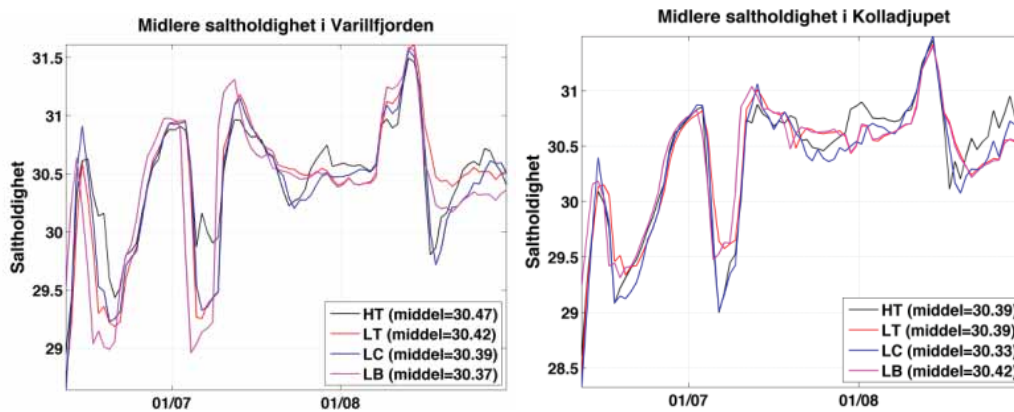
Figur 28. Som i Figur 27, men tidsutviklingen av saltholdighet er vist.
