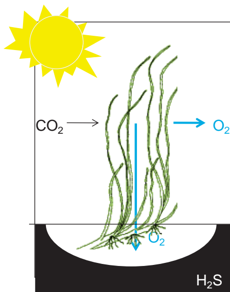
Figur 3. Ålegresset tar opp karbondioksid ( CO_2 ) fra vannet skiller ut oksygen ( O_2 ) gjennom primærproduksjonen til va bunn-sedimentet.
