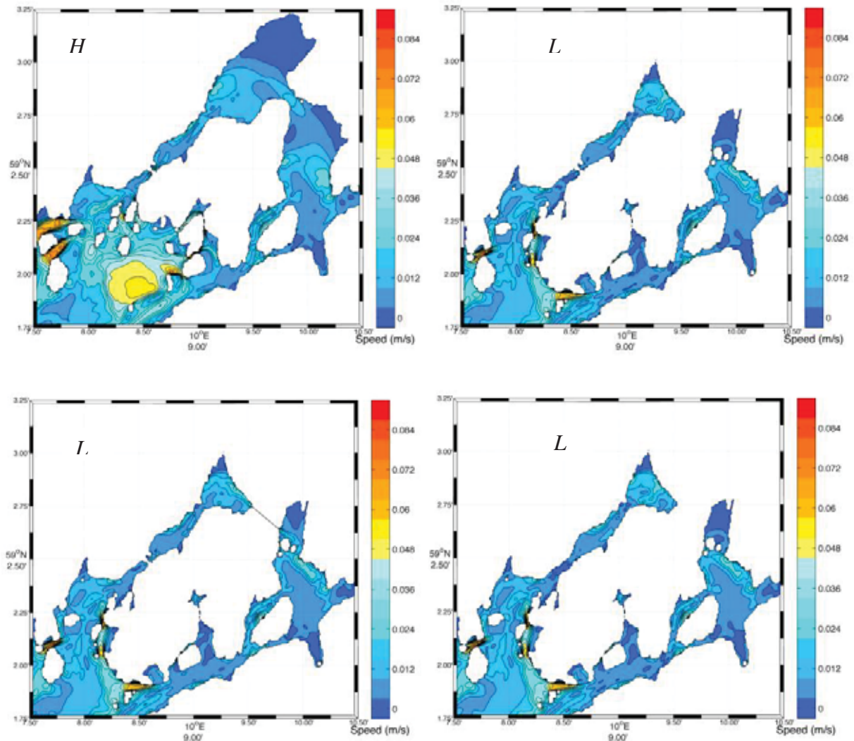
Figur 22. Gjennomsnittlig, dybdeintegret strømhastighet (i m/s) over ca. 2,5 måneder (juni-august) for scenariet med høyvann (HT), lavvann (LT), lavvann og åpning av kanal innerst i fjorden (LC) og med lavvann og fjerning av brua over til Vikerøya (LB).
