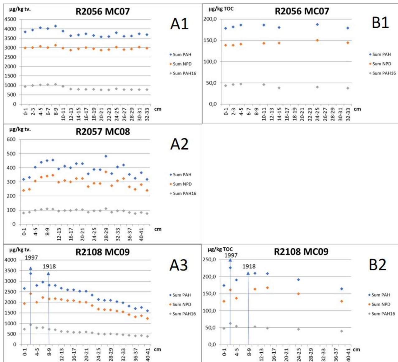
Figur 11. Dybdeprofiler av Sum PAH, NPD og PAH16 i sedimentkjerner fra Kongsfjorden. A: PAH-nivåer i \mu\text{g}/\text{kg tv.} ; B: PAH-nivåer korrigert for TOC. Ca. årstall er vist for to snitt i den daterte kjernen.
