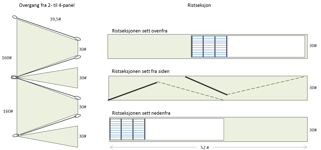
Figur 12: Firepanel fleksiristseksjon med overgang fra to- til firepanel (Tegning: Eduardo Grimaldo & Manu Sistiaga).
