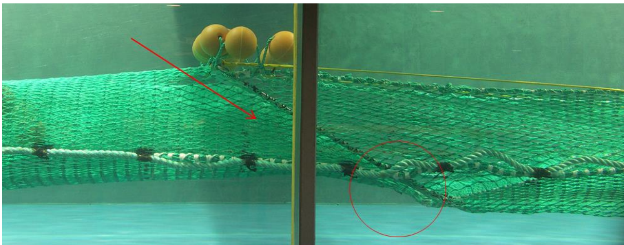
Figur 6. Bilde av 2-panel ristseksjon som viser hvordan løftepanelet legger seg inntil rista og blokkerer den, og hvordan hovedseksjonens underpanel også presses opp foran og inntil rista (Gjørund et al., 2013).
