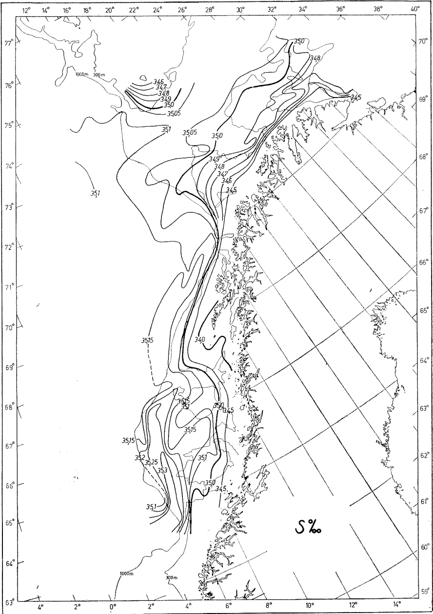
Fig. 5. B) Salinity at 50 m.
