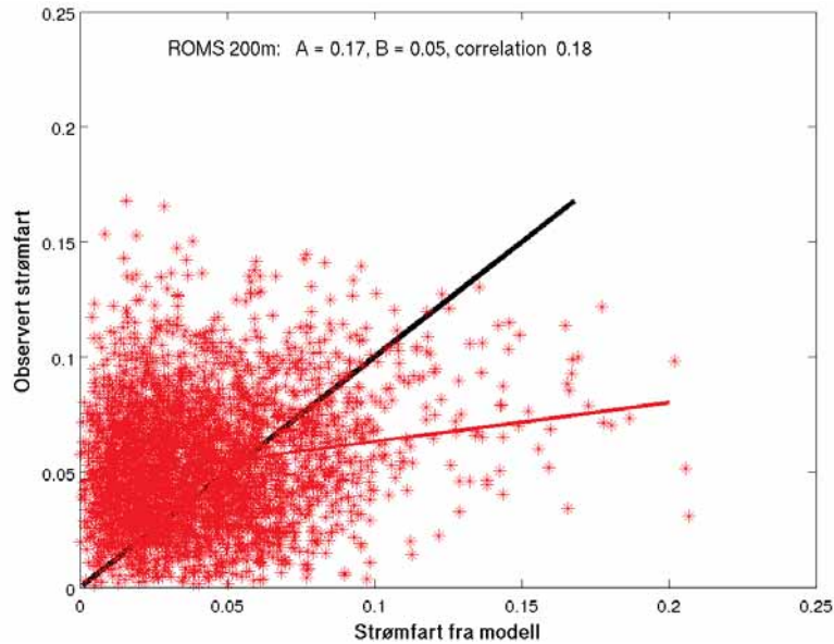
Figur 18. Målt og modellert strømfart fra st. 2 (nordøstlige) i alle nivåer mellom 10 og 30 m mellom 15. april og 14. mai 2009 er plottet mot hverandre, og hver verdi er angitt med en rød stjerne. Modellverdi er angitt langs horisontal-aksen og målt verdi langs vertikalaksen. Den svarte linjen angir 1:1 forholdet mellom måling og modell, mens den røde linjen er en enkel lineær regresjonslinje fra de aktuelle punktene. Korrelasjonsfaktoren mellom observasjoner og modellverdier er i dette tilfellet 0.18.
