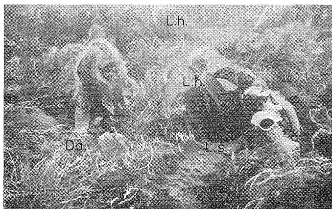
Fig. 8. Blandet vegetasjon av stivt kjerringhår ( Desmarestia aculeata = D.a.), sukkertare ( Laminaria saccharina = L.s.) og stortare ( L. hyperborea = L.h.) etter 3 års gjenvækst. Dybde 8 m. Bøskinnene, den 24. august 1970. [Mixed vegetation consisting of Desmarestia aculeata = D.a., Laminaria saccharina = L.s. and L. hyperborea = L.h. growing at 8 m depth in an area harvested 3 years previously].
