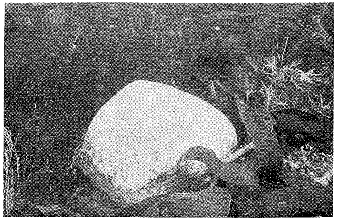
Fig. 6. Virkning av stortaretrål på stenbunn. Stenen som anslagsvis veier mellom 1 og 1,5 tonn er veltet helt rundt. Dybde 8 m. Bøskinnene, den 24. august 1970. [Effect of a large seaweed dredge on stony bottoms demonstrated by the overturned boulder with an estimated weight of 1–1,5 tons. Depth 8 m.]
