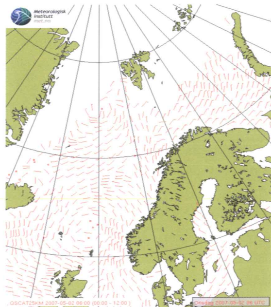
Figur A.3.10. Eksempel på vindsituasjonen i Norskehavet basert på QuikSCAT satellittbilde. Vindpilene viser vindstyrke og -retning 10 m over havflaten. Vindretningen er vist ved piler. Vindstyrken er angitt som faner på pilene, halv fane er 5 knop (ca. 2.5 m/sek, Bf 2), hel fane er 10 knop (ca. 5m/sek, Bf 3) og flagg er 50 knop (25.7m/sek, Bf 10). Figur fra www.oljedirektoratet.no .
