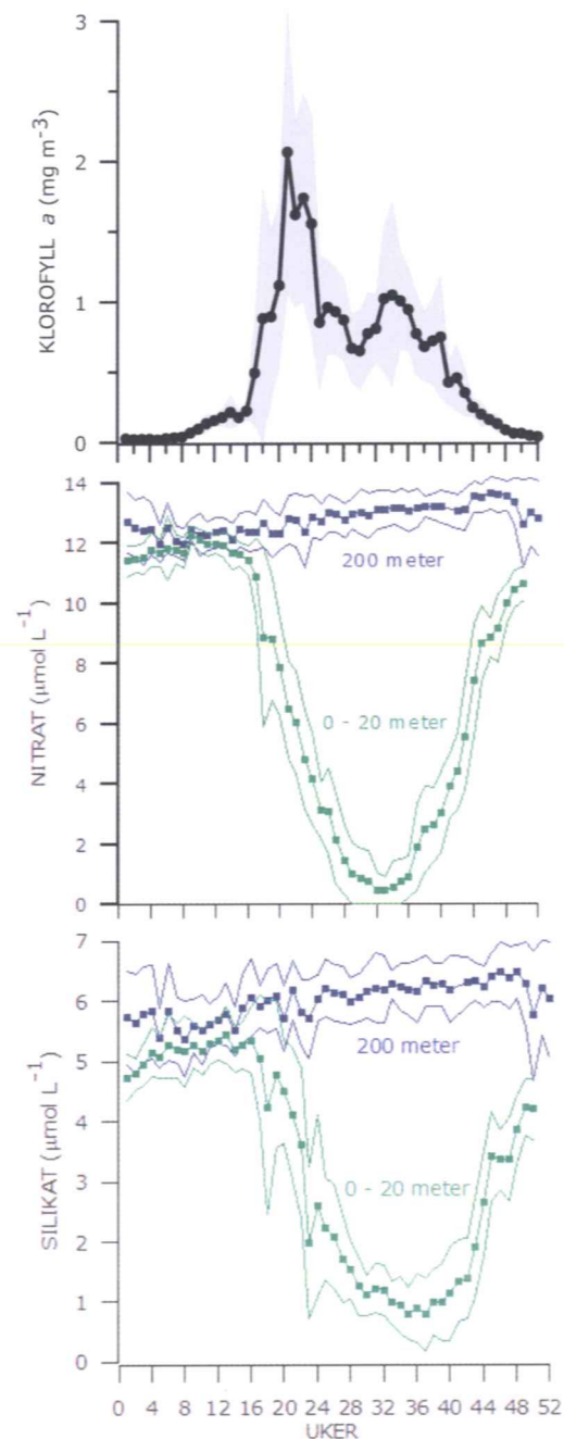
Figur A.4.4. Sesongmessig fordeling ved Værskipstasjon Mike ("Stasjon M", 66° N; 02° Ø), av A) klorofyll a ( \text{mg m}^{-3} ), B) nitrat ( \mu\text{mol l}^{-1} ) og C) silikat ( \mu\text{mol l}^{-1} ) i de øverste 20 meter og ved 200 meter dyp. Punktene viser gjennomsnitt verdier for perioden 1990-2006. De tynne linjene viser standardavvikene. Kilde HI.
