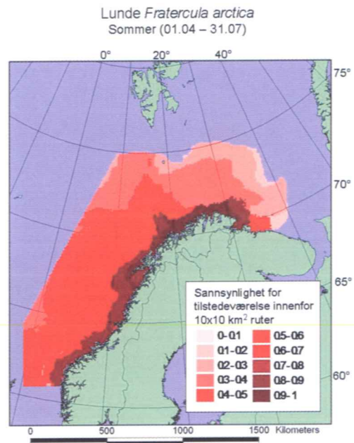
Figur A.9.4. Lunde. Til venstre: Lundepar © Jo Anders Auran. Til høyre: Modellberegnet utbredelse for lunde Fratercula arctica i sommersesongen. Utbredelsen er en kombinasjon av at fuglene er knyttet til koloniene på land og at de finner næring langs kysten (SEAPOP 2007).
