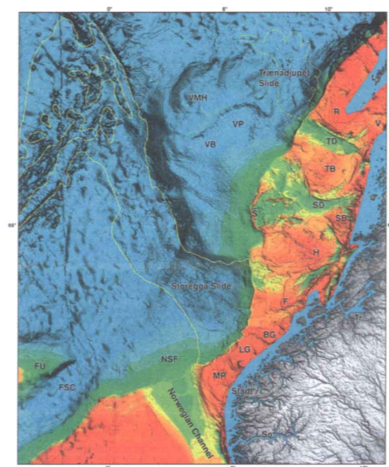
Figur A.2.2. Oversikt over midt-norsk sokkel, kontinentalskråningen og dyphavet innenfor deler av forvaltningsplanområdet. Storeggaraset og Trøndjupraslet er inntegnet med gul strek. VP=Vøringplataet. Datagrunnlag: Statens Kartverk, Sjøkartverket. Figuren laget av Dag Ottesen, NGU.
