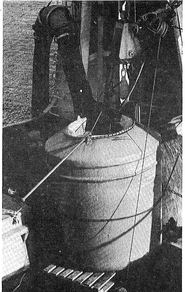
Fig. 11. Filtrering av sjøvann fra fiskepumpen. Vannet siles gjennom en håv som står i vannbad på dekk.
