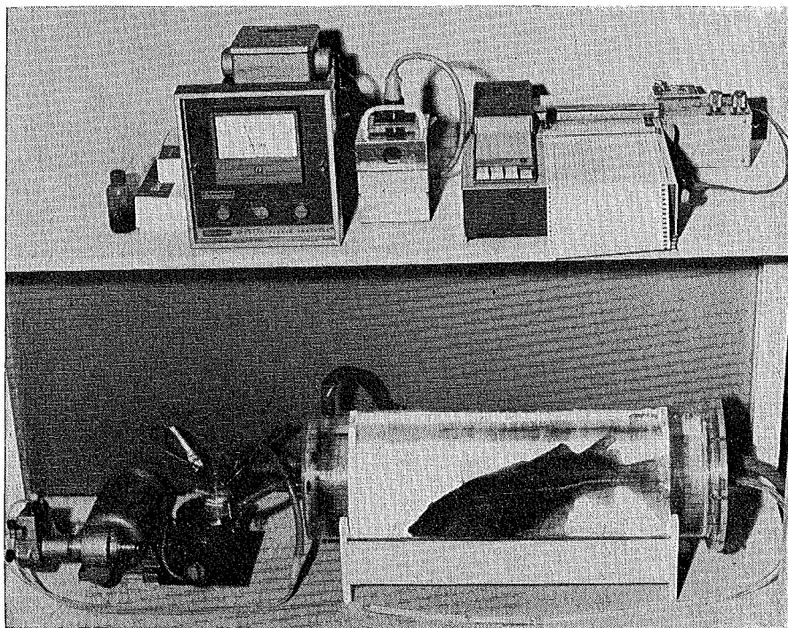
Fig. 6. Apparat for måling av stoffskifte hos fisk. (Foto: G. Monsen.)
