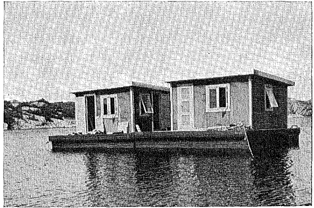
Fig. 7. Feltstasjon for undersøkelser over virkning av støy på fisk. (Foto: K. Olsen.)
