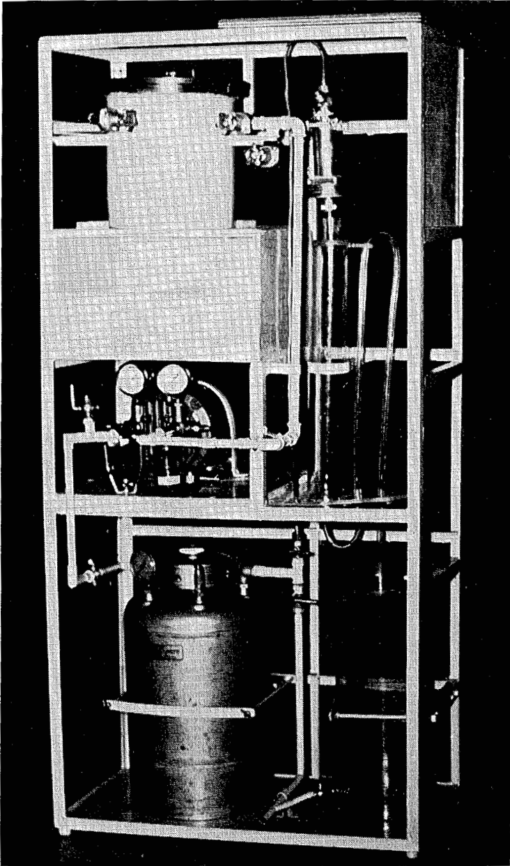
Fig. 1. Apparat for filtrering av sjøvann for klorofyllbestemmelse. (Foto: G. Monsen.)
