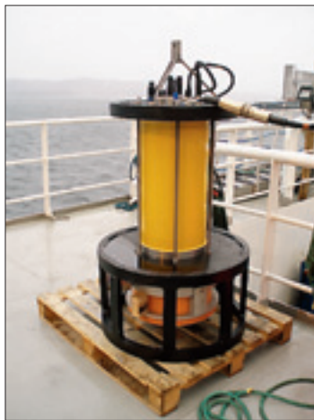
VIKTIG: En TS-probe brukes til å finne ut hvordan lodda reflekterer energi som sendes ut fra ekkolodd, og er et meget viktig instrument i vinterens loddeundersøkelser
