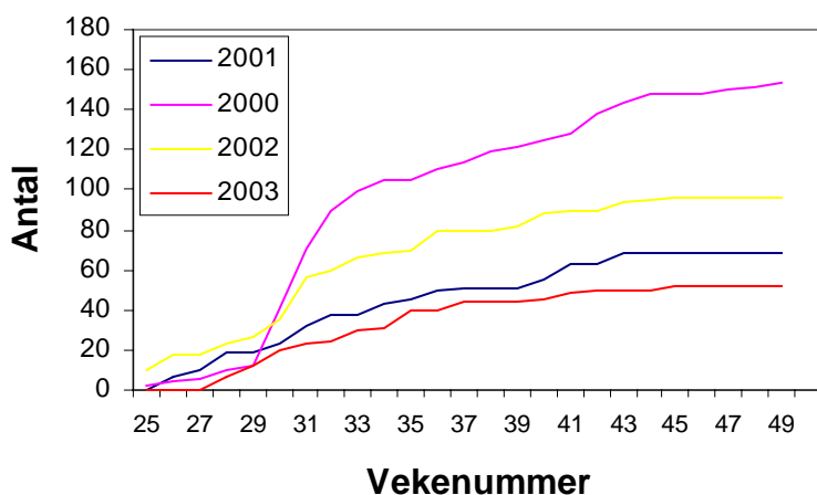
Figur 20. Oppvandra vill sjøaure i Guddalselva 2000-2003. Ein indikator på sjøoverlevinga i midtre del av Hardangerjorden.
