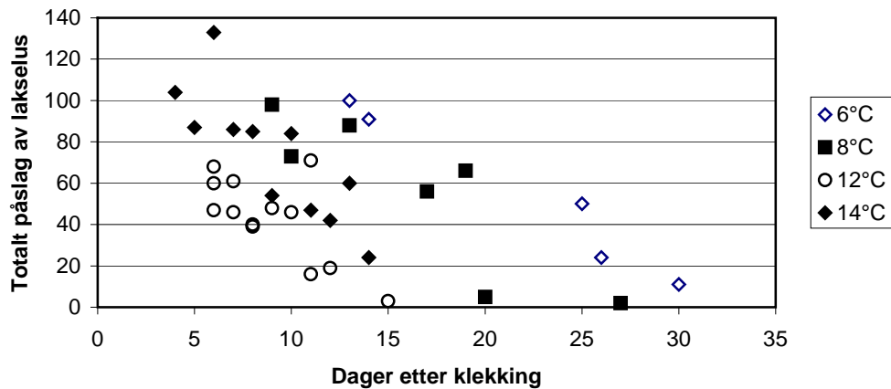
Figur 26. Påslagssuksess av lakselus ved ulike temperaturer og med copepoditter av økende alder (Boxaspen, in prep).
