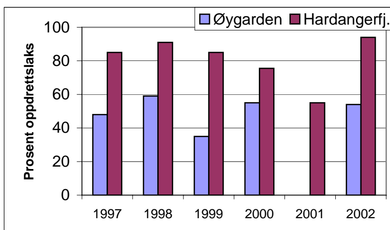
Figur 14. Andel oppdrettslaks i sjøfisket etterlaks i Øygarden og Hardangerfjorden 1997-2002. (NINA, 2001).
