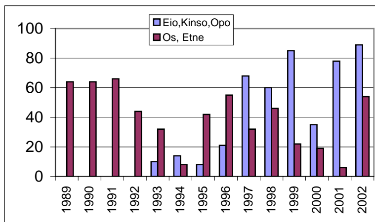
Figur 15. Andel oppdrettslaks i elvar i indre Hardangerfjorden (Eio, Kinso og Opo) og i ytre deler (Etne og Os). Tala viser at variasjonen er stor mellom år, og at problema med rømt fisk oppstod tidlegare i ytre område enn i dei indre områda av Hardangerfjorden. (DN rapport 2001-2).
