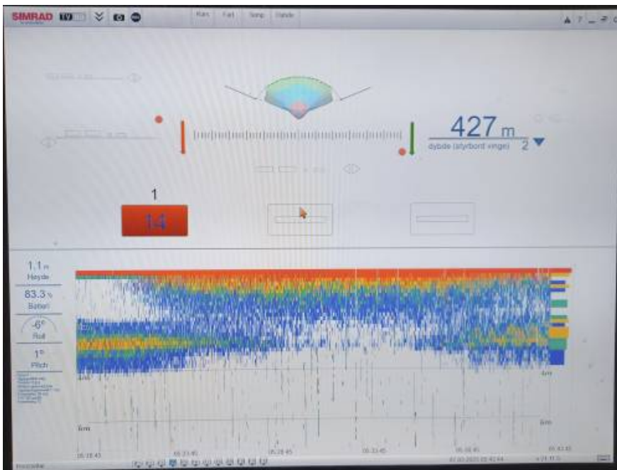
Bilde 13. Bilde fra tråloye montert bak på fangstbegrensningsseksjonen. Vi ser bunnen på seksjonen 3 m under toppanel. Bunnen registreres ikke når fisketettheten er størst.
