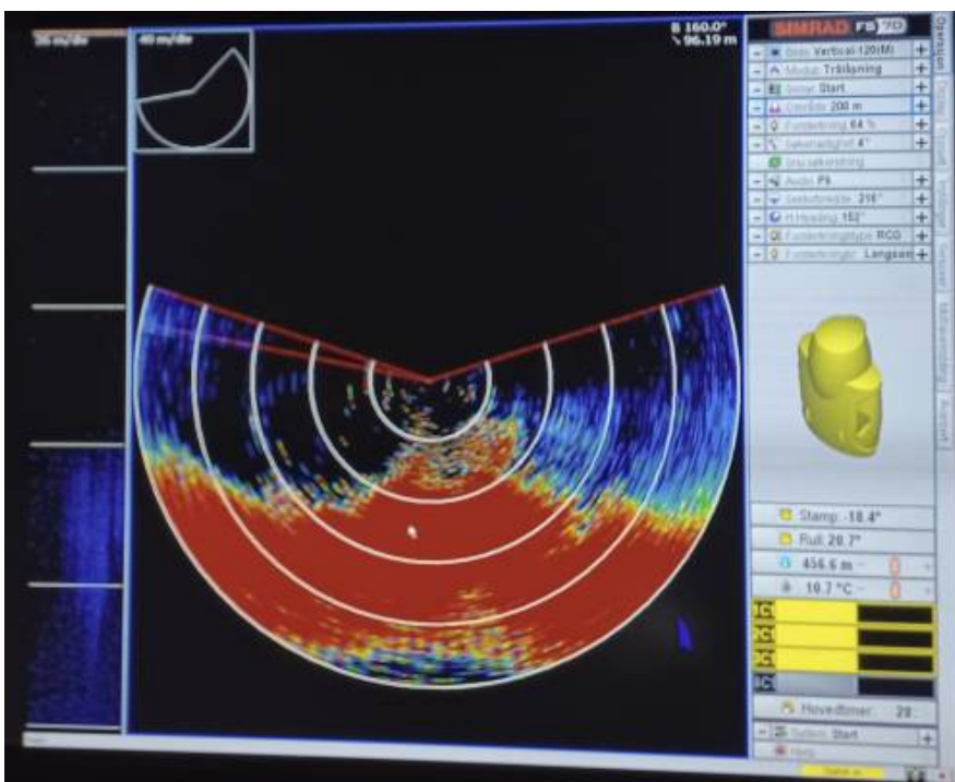
Bilde 14. Bilde fra trålsonar. Det er ikke lett å se trålen, høyden har vi estimert til ca. 130 m (litt mer enn de tre innerste ringene).
