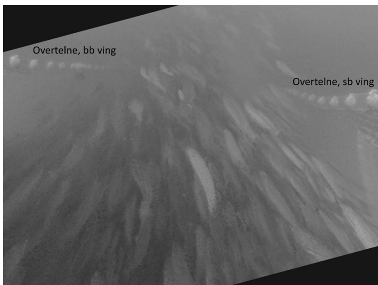
Figur 12. GoPro video fra overtelne, kast 2. Figur til høyre viser kameras plassering og orientering.
