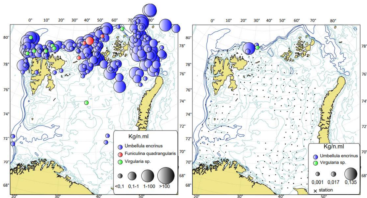
Figur 4.1.4.6 Biomasse-fordeling (kg/n.ml) av sjøfjær i Barentshavet i henhold til Økosystemtoktet 2005–2020 (venstre) og i 2021 (høyre) De svarte punktere angir stasjonsdekning. Stasjoner i nord-russisk sone og det sentrale Barentshavet manglet i 2021. Kilde: ICES (2022d).
