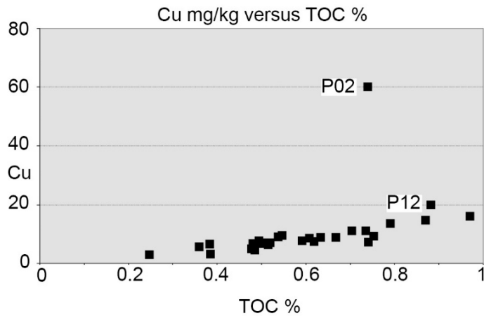
Figur 3.9. Nivåer av kobber (Cu) i overflatesedimenter plottet mot totalt innhold av organisk karbon (TOC).
