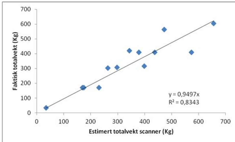
Figur 1 Telleresultater scannet totalvekt i forhold til faktisk totalvekt fra alle testene av AquaScan, bortsett fra simuleringene fremstilt grafisk. Hvert punkt indikerer en test, og avstand fra trendlinjen angir avvik fra fasit.
