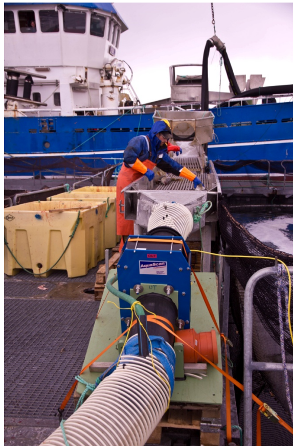
Bilde 5 Bildet viser test av AquaScan under levering av levende torsk til merd fra snurrevadbåten MS Kildin.
