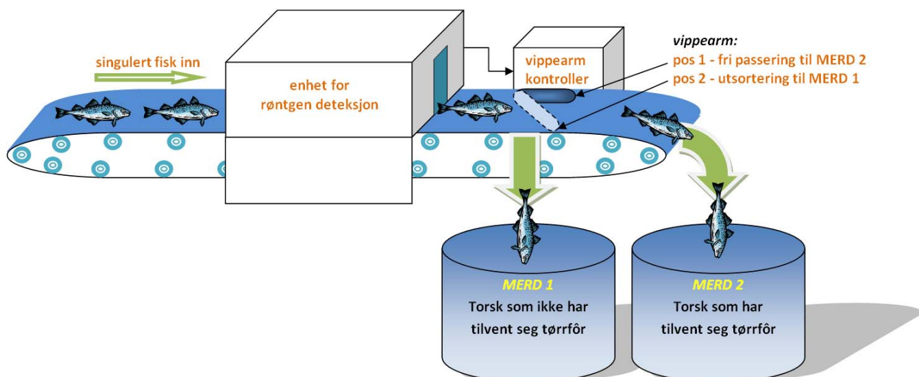
Figur 28 Skisse av helhetlig linje for sortering, med transportband og vippearms / sorterer montert (Illustrasjon: Emil Veliyulin). Formål er sortering av fisk basert på fettinnhold i fôr.
