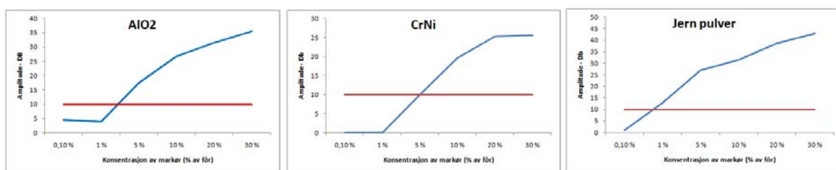
Figur 25 Eksempler på følsomhet til metalldetektor ved metaller og partikkelstørrelser. Rød linje viser deteksjonsgrense.
