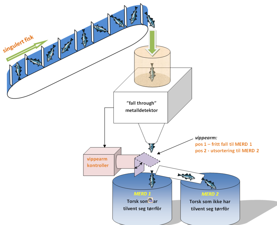
Figur 29 Skisse av linje som sorterer fisk basert på metalledeksjon. Fisken må føres med pellets til satt partikler for øke kontrasten (Illustrasjon: Emil Veliyulin). Formålet er sortering av fisk basert på deteksjon av metaller i fôr.
