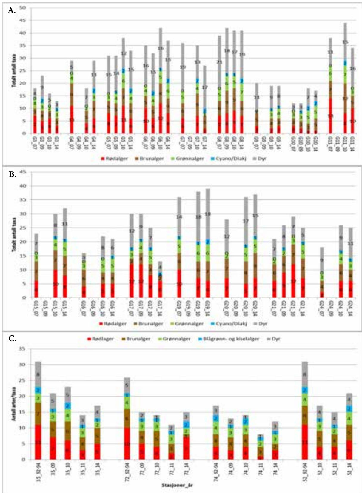
Figur 27. Fordelingen av antall arter/taxa av rød-, brun- og grønnalger, blågrønnalger/kiselalger og dyr registrert på de 16 rammestasjonene og 4 strandsonestasjonene som ble undersøkt i 2014. A. Rammestasjonene på vestsiden av Oslofjorden. B. Rammestasjonene på østsiden av Oslofjorden. C. Strandsone-stasjonene i Hvalerområdet (undersøkelser for Borregaard AS).
