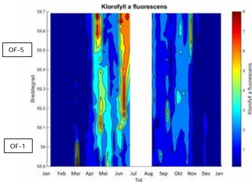
Figur 14. Konturplott av klorofyll a fluorescens på 4m dyp i 2014. Data er vist for området fra grensen mot svensk farvann og opp til Drøbak. Data fra Ferrybox.
