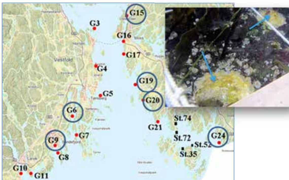
Figur 24. Kartet viser plassering av hardbunnstasjoner i strandsonen i 2014. Ramkestasjonene er merket med røde sirkler. Det ble i tillegg foretatt strandsonundersøkelser ved 4 stasjoner, merket med sorte firkanter. Den fremmede arten stillehavsøsters (se blå pil på innfelt foto) ble observert ved stasjoner markert med blå sirkel. Foto fra stasjon G20.
