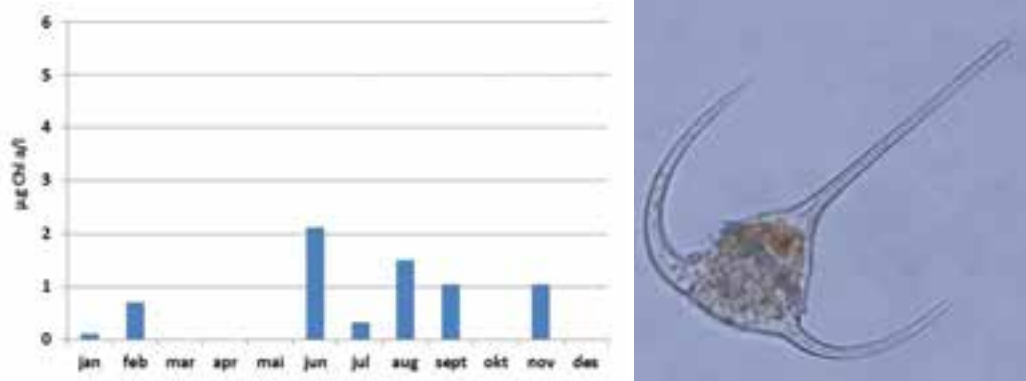
Figur 18. Mengden klorofyll-a ( \mu\text{g Chl a/l} ) ved stasjonen «Torbjørnskjær» OF-1 ytterst i Oslofjorden i 2014. Dinoflagellaten Ceratium tripos (bilde) var den dominerende arten i slekten Ceratium i Oslofjorden i 2014. Foto: Havforskningsinstituttet.
