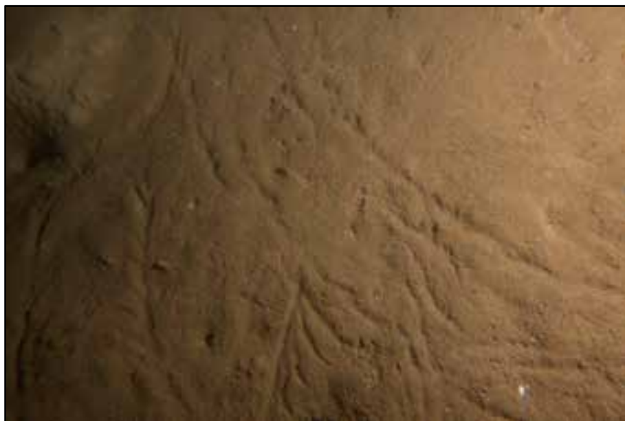
Figur 22. Torbjørnskjær (OF-1) 450m dyp. Klassifisert som 'god' bentisk habitat (i hht BHQ-indeks). Sedimentoverflaten har brunlig farge, og er dekket av nylig sedimentert organisk materiale. På overflaten ser man spor av dyr som har beveget seg oppå sedimentet, og også noen få hull fra bløtbunnsorganismer som lever nede i sedimentet (antakelig børstemark og muslinger).
