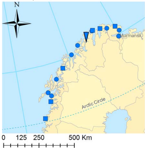
DDT i blåskjell
