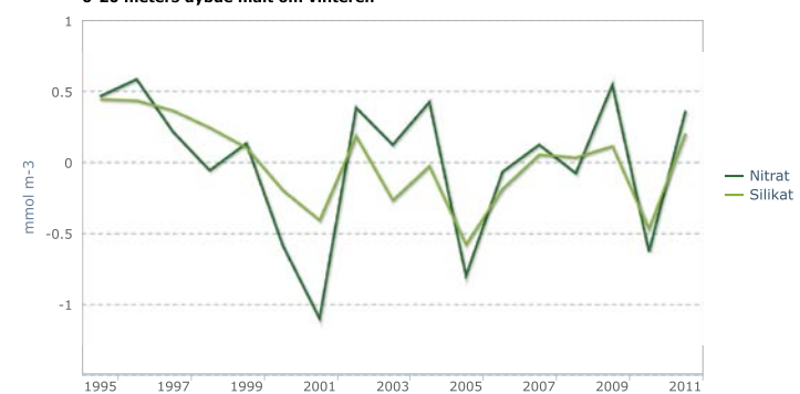
Avvik i konsentrasjon av nitrat og silikat i kystvann 0-20 meters dybde målt om vinteren
