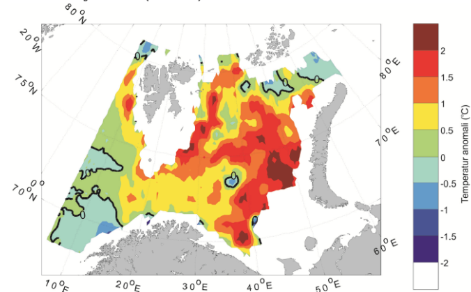
→ Temperaturavvik i 100 m dyp i august-september 2012 i forhold til langtidsmiddelet (1977-2006)
