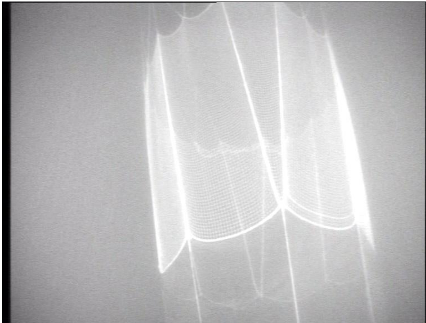
Figur 15. Trålbelt av kvadratmasker og med ekstra over- og underpanel (trekantfasong).
