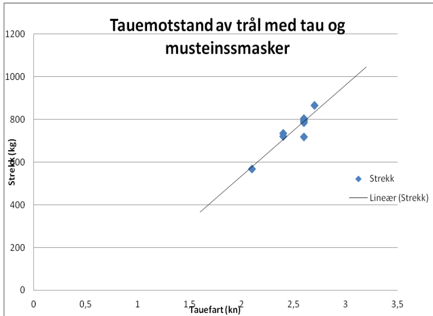
Figur 14. Motstand til trålen laget av tau og mursteinsmasker med varierende tauemotstand.
