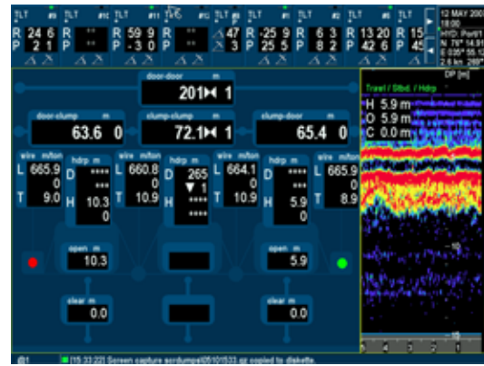
Figur 8. Scanmar målinger fra hal 13 (samtidig med bilde i Figur 6). Trårløye bildet er fra den eksperimentelle trålen.
