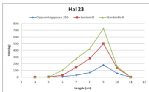
Figur 14. Fangstfordeling av reke i kg i eksperimentell trål og standard trål, samt beregnet tap av ulike reke-størrelser gjennom sidepanelene i hal 23.
