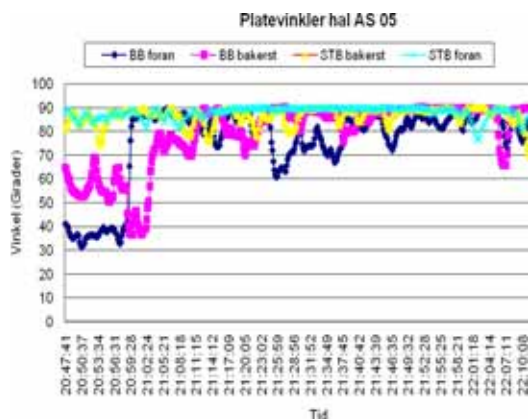
Figur 9. Platevinkler målt på 4 plater langs gearet i hal AS 05. 0^\circ = Vertikale plater og +90^\circ =horisontale plater.
