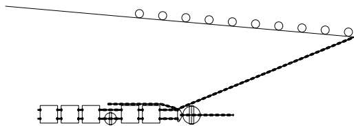
Figur 10. Rigging av vingespisser på den eksperimentelle trålen utstyrt med plategear langs vingene.
