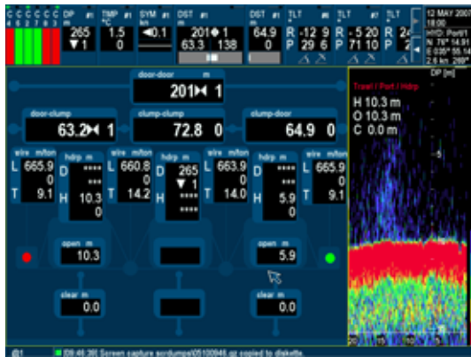
Figur 7. Scanmar målinger i hal 13. Trårløye er montert på standard trål på babord side.
