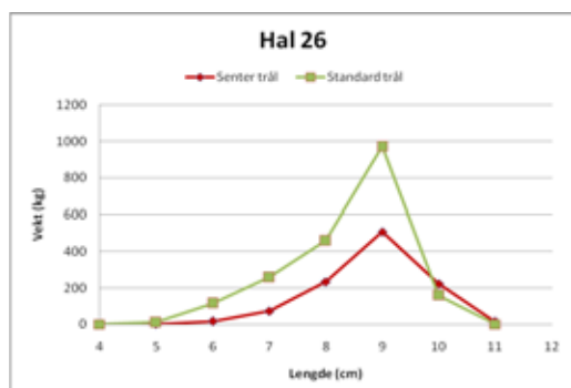
Figur 16. Fangstfordeling av reke i kg i eksperimentell trål og standard trål i hal 26.
