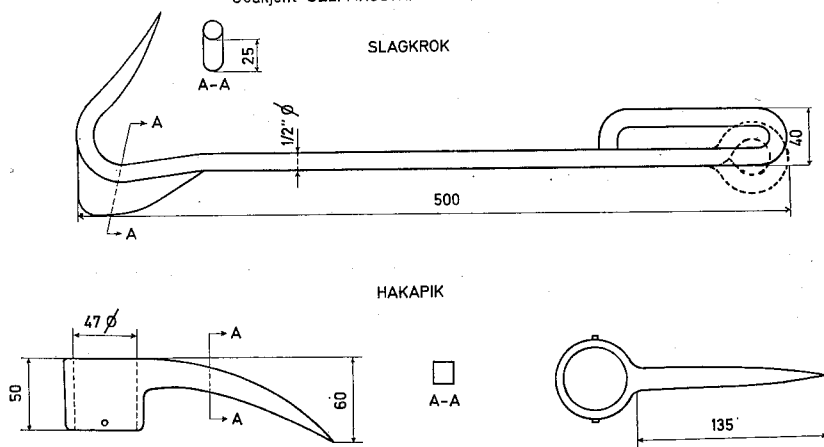
Figur 1. Typetegninger for slagkrok og jernsko til hakapik. Slagkroken skal være 50 cm lang, veie minst 800 gram medregnet den påsveide tilleggsvikt ved kroken, og skal lages av halvtoms rundjern, kvalitet ST-37-D. Håndtaket kan utformes som øye. Viklinger vil gi bedre grep. Jernskoen til hakapiken skal også lages av smijern, kvalitet ST-37-D, og skal veie minst 400 gram. Den bøyde piggen kan være fra 12 cm til 18 cm lang. Jernskoen kan også påsveies en hammertapp som ikke må være mer enn 4 cm lang. Jernskoen skal være forsvarlig festet til et rett skaft laget av bjerk. Skaftet kan være fra 110 cm til 150 cm langt, og skal ha en diameter på fra 3 cm og til 5 cm.
