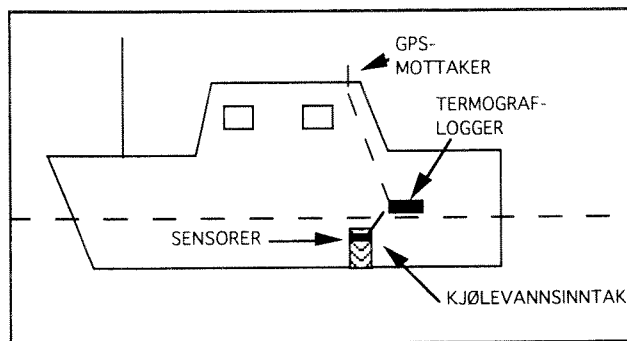
Montering av termograflogger i leilighetsskip
