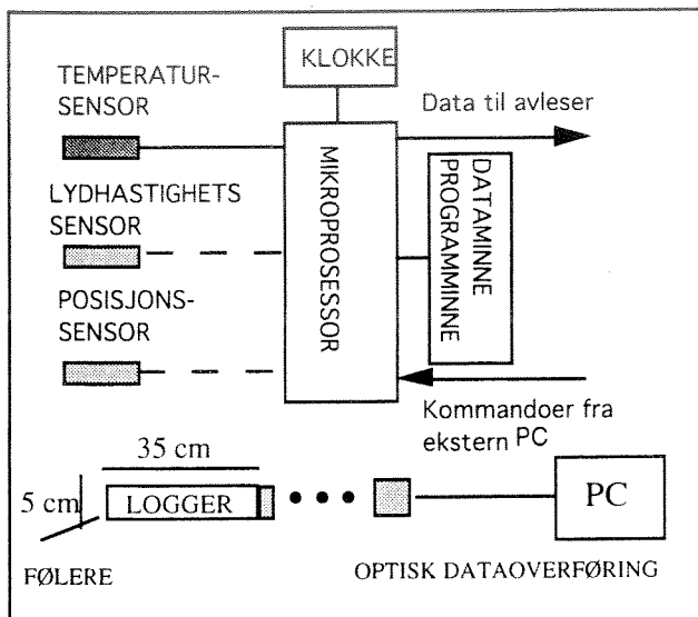
Prinsipp for moderne termograflogger
