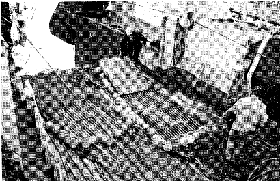
Fra utprøvinga av SortV-rista (t. v.). Til høyre ser vi Sortx-rista.
