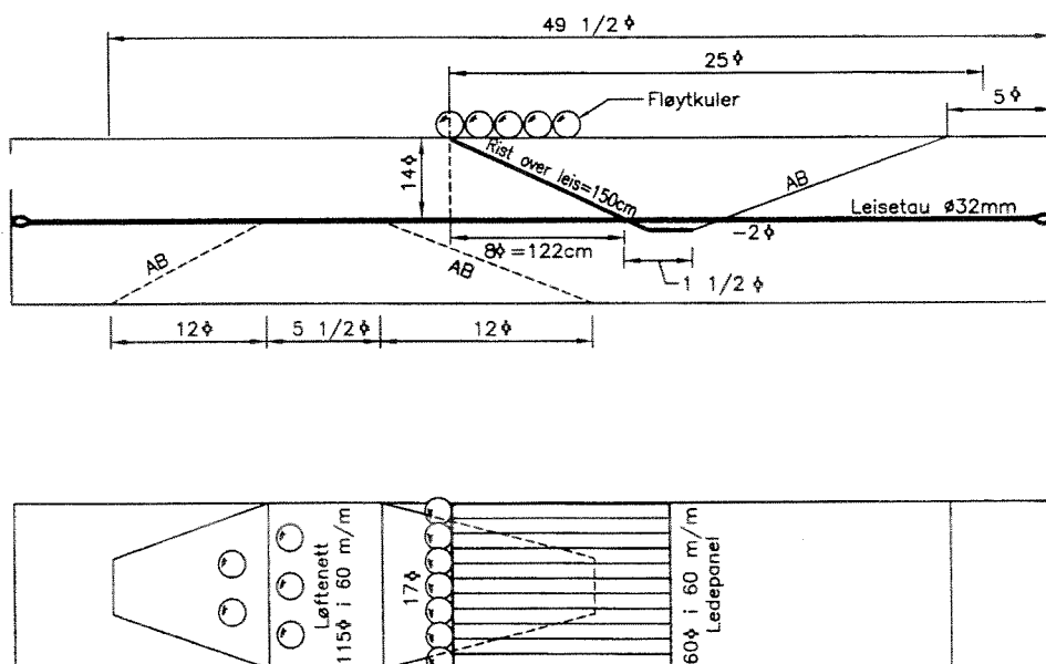
Teknisk tegning av SortV-rista montert i trål. Øverst er rist sett fra siden. Nederst ser vi den fra oversiden.
