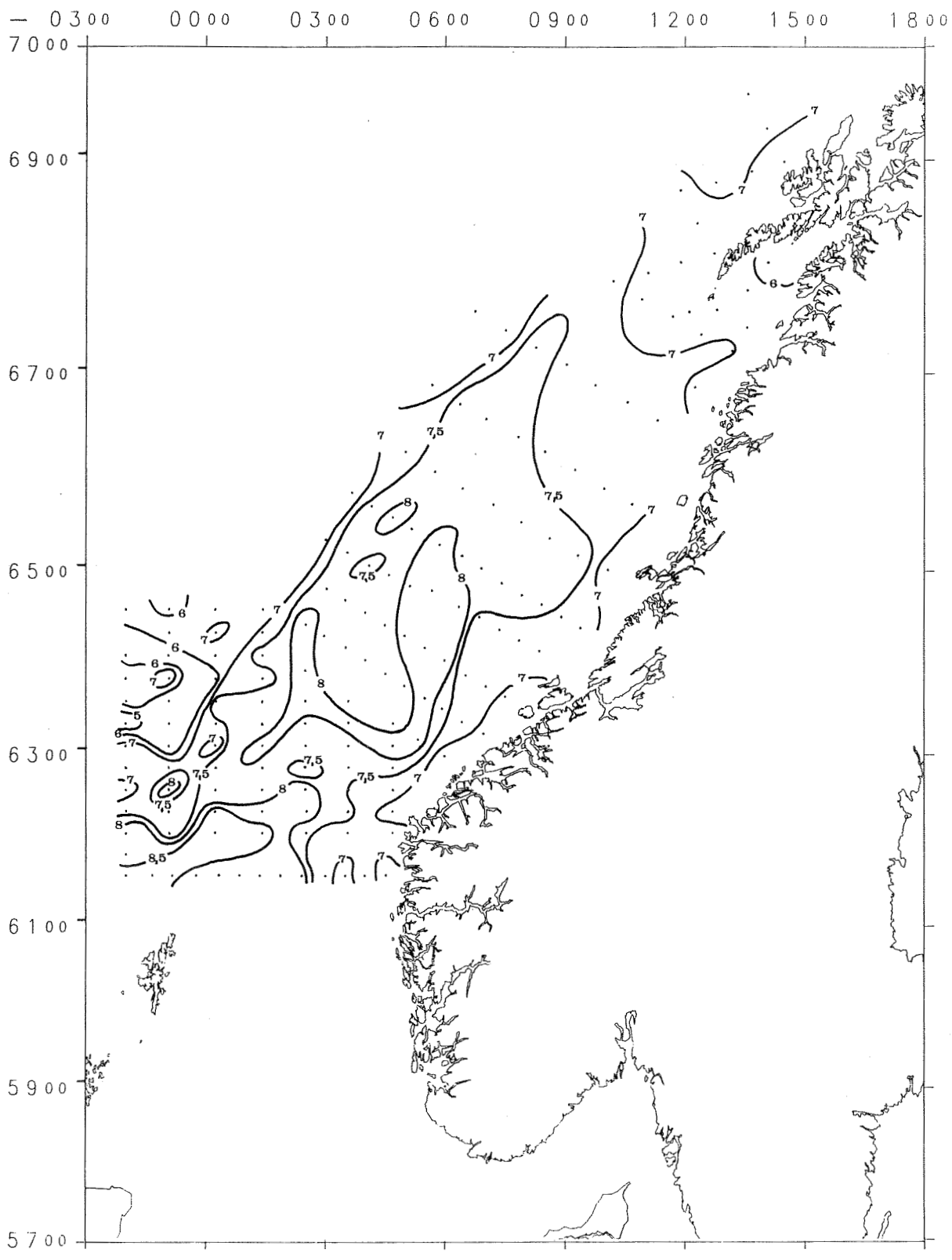
Figur 8. Fordeling av temperatur ( ^{\circ}\text{C} ) i 50 meters dyp ("Eldjarn").
