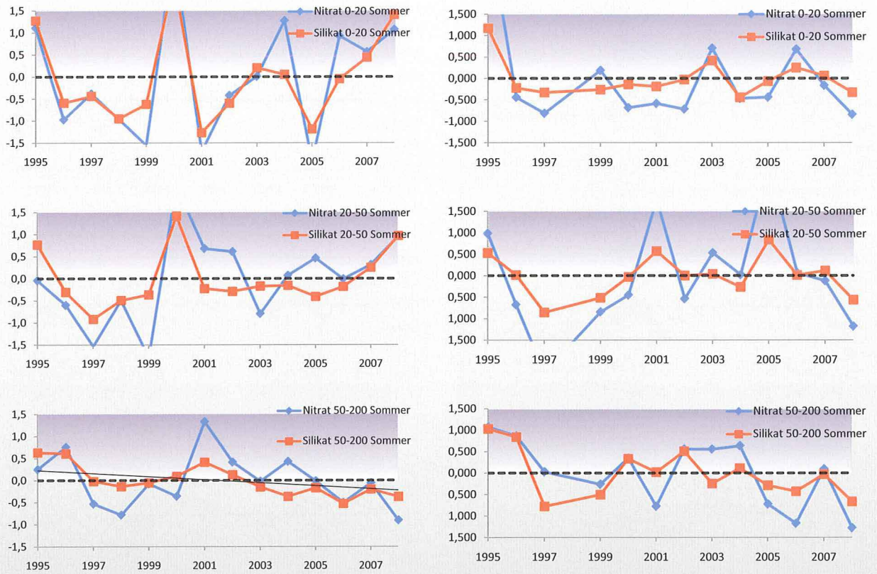
Figur 4.1.2.5 Avvik i konsentrasjoner av nitrat og silikat om sommeren i tre dybdelag i Atlanterhavsvannet i snittene Fugløya-Bjørnøya og Vardø-nord i perioden 1995 – 2008.
