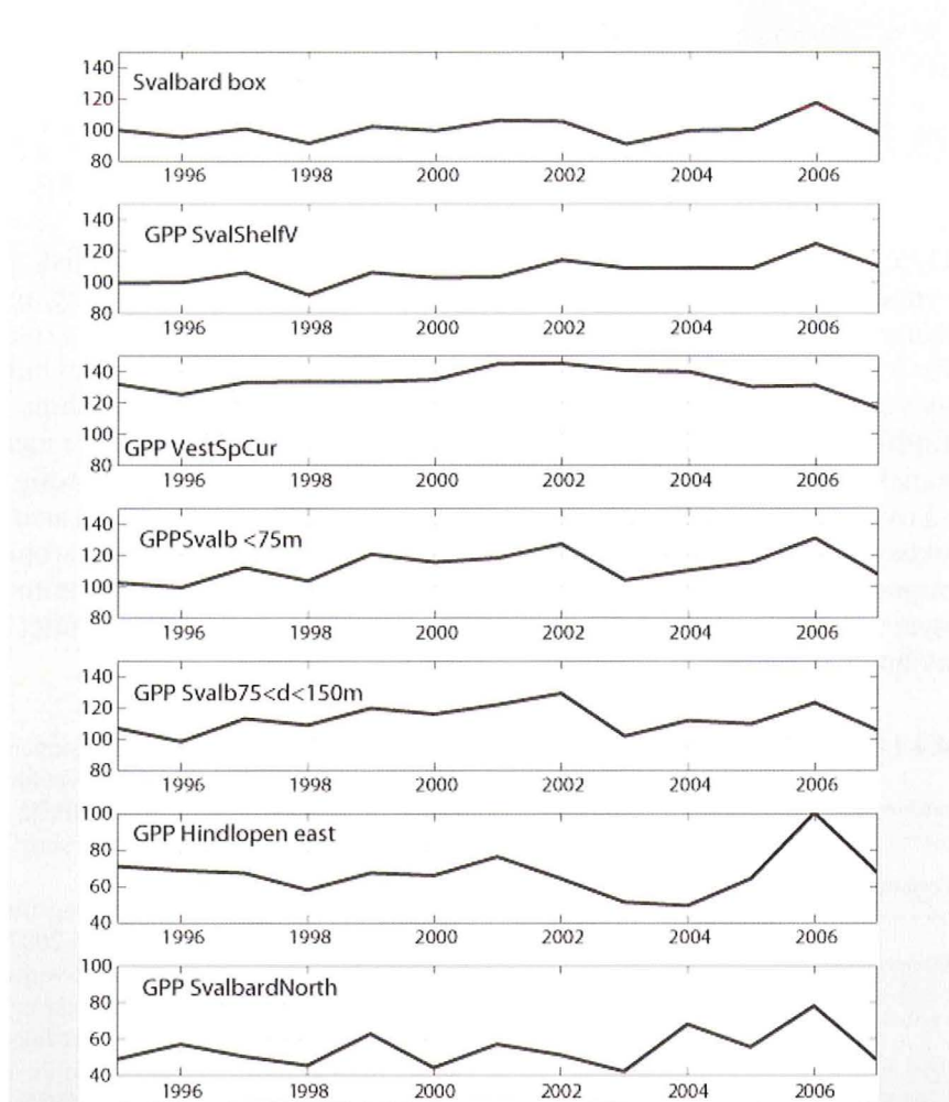
Figur 4.3.2.5 Modellert primærproduksjon (g C m -2 ) for delområder av Barentshavet i perioden 1995-2007. Merk at skalaen på Y-aksen er ulik mellom figurene. Delområdene er: Svalbard box – "Svalbard sektor", 0 – 40 °E, 74 – 82 ° N; SvalShelfV – Sokkel vest for Svalbard og Storfjorden; VestSpCur – Vest Spitsbergenstrømmen; Svalb<75m – Svalbardbanken dyp mindre enn 75 m; Svalb75<d<150m – Svalbardbanken, dyp mellom 75 og 150 m; Hindlopen east – Hindlopen til 40 °E; SvalbardNorth – Svalbard til 82 °N.
