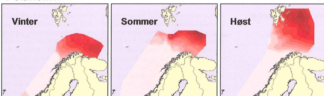
Figur 4.8.1.2 Sesongforflytninger: Fordeling av lunde og polarlomvi i Norskehavet og Barentshavet i ulike sesonger.
