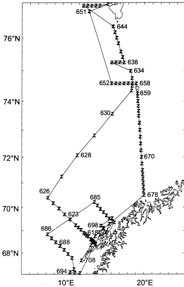
30 Jun - 21 Jul 1998 z CTD st.no 608-709 "Michael Sars" Cruise no 1998108 Standard sections Gimsøy NW st.no 608-626 Fugløya - Bjørnøya st.no 659-678
