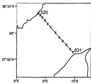
7-8 Dec z CTD st.no 520-531
