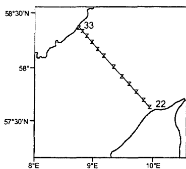
24 Feb z CTD st.no 22-33
