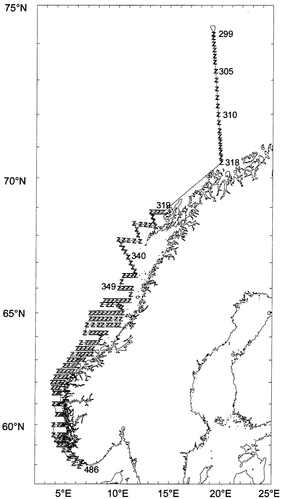
6 - 24 April 1998 z CTD st.no 299-486 "Michael Sars" Cruise no 1998104 Standard section Fugløya- Bjørnøya: st.no 299-318
