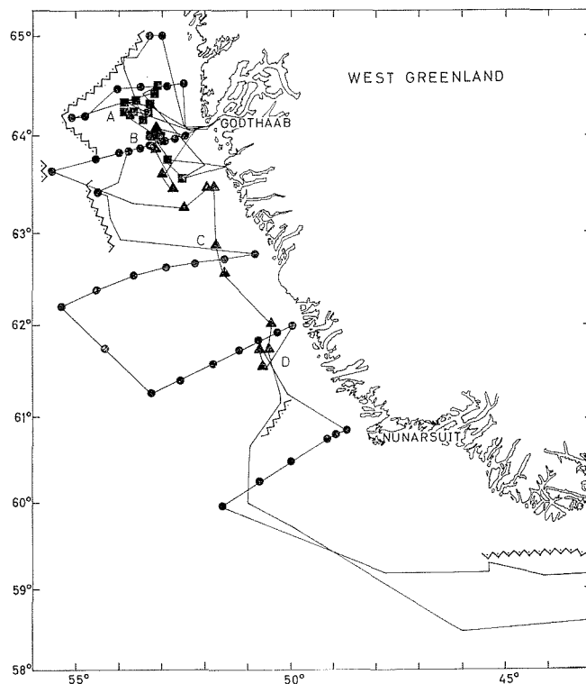
Fig. 1. «Johan Hjort», Vest-Grønland, april/mai 1964. Kurser og stasjonsnett. ● : hydrografiske stasjoner, ▲ : linestasjoner, ■ : trålstasjoner, AAA : isgrense. A: Bananbanken, B: Fyllas bank, C: Danas bank, D: Navnløsebanken.
