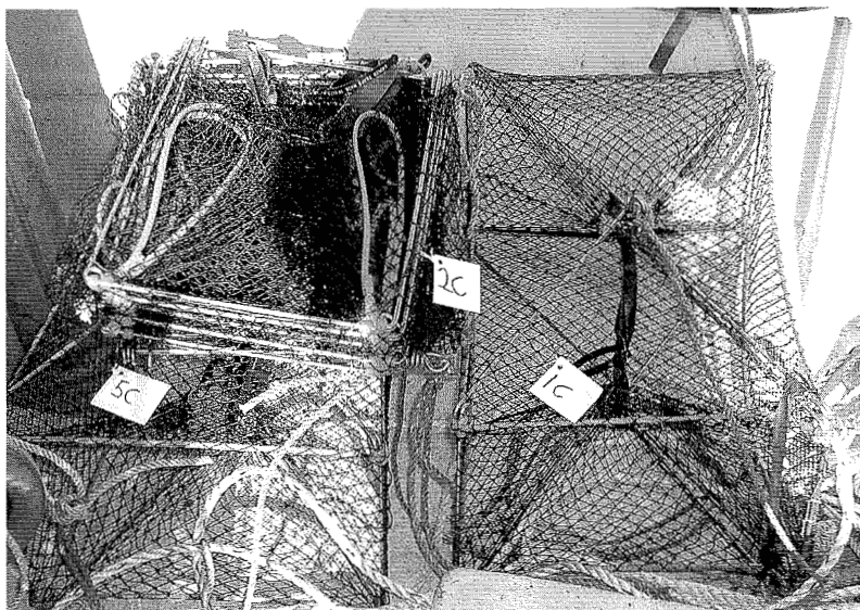
Figur1: Reketeinene brukt i forsøksfisket i Tanafjorden; a) type A teine (Stealth shrimp pot), b) type B teine (Ladner heavy shrimp pot) og c) type C teine (Ladner folding prawn pot).
