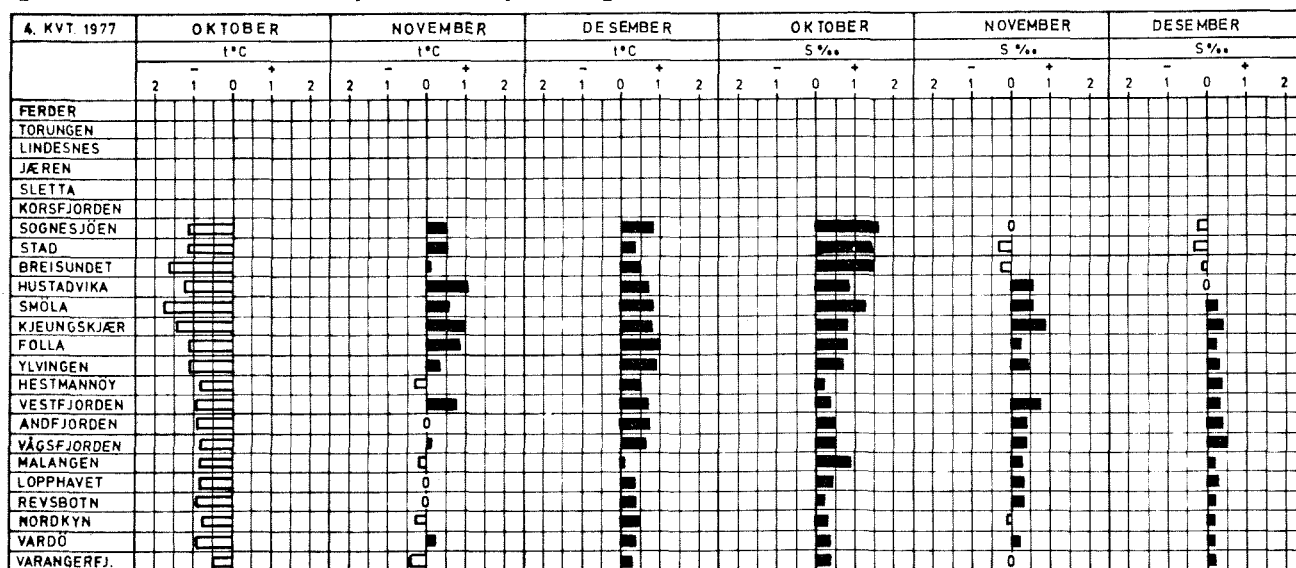
10 dagers middeltemperatur og månedsmiddel for saltholdighet langs Norskekysten i 4. kvartal 1977.
