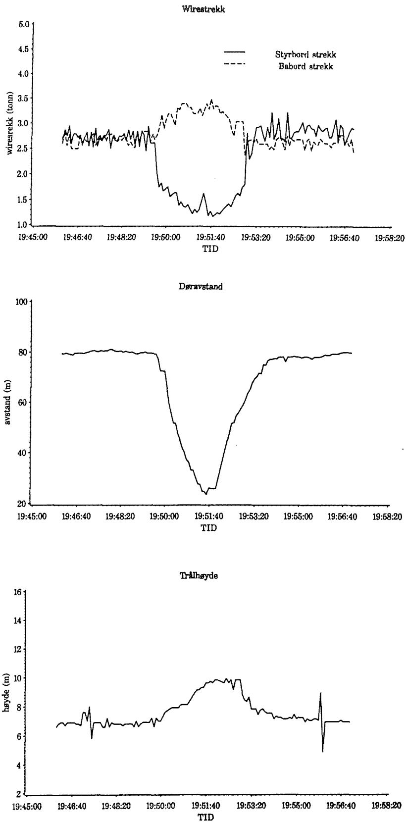
Figur 15. Strekk og geometri av Expo 1200 m/gear ved 18^{\circ} krysningsvinkel og der tråldøren reiser seg straks etter rørplassering [Tension and geometry of the Expo trawl, 1200 meshes with gear, at a 18^{\circ} crossing angle, where the trawl door raises immediately after having crossed the pipeline].
