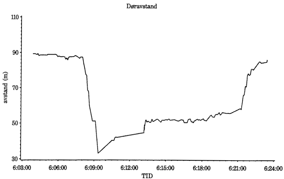
Figur 19. Strekk og geometri av Expo 1200 m/sabb med 18^{\circ} krysningsvinkel der tråldøren ligger med baksiden ned i ca. 10 min. etter rørpasering (MS 30, 3. krysning) [Tension and geometry of the Expo trawl, 1200 meshes with gear, at a 18^{\circ} crossing angle, where the trawl door is lying backside down for about 10 minutes after having crossed the pipeline (trawl station no. MS 30, third crossing)].
