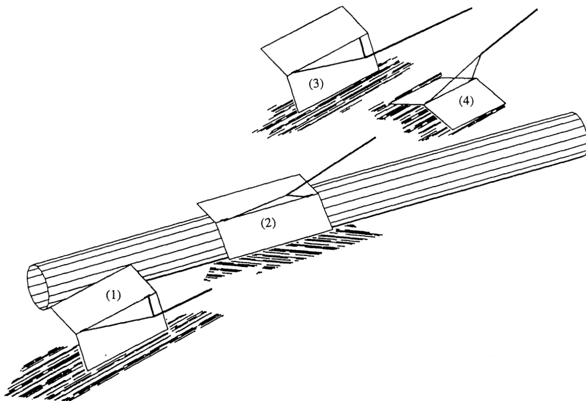
Figur 14. Skjematisk illustrasjon av hvordan en tråldør som treffer rørledningen med lave innfallsvinkler oppfører seg når den følger røret og etter at den er dradd over. 1) Tråldøren normalt operativ før den treffer rørledningen, 2) tråldøren trekkes langs rørledningen liggende med baksiden mot røret, 3) tråldøren har passert røret og er oppreist, og 4) tråldøren har passert røret og ligger med baksiden ned [ Schematic illustration of the performance of a trawl door hitting the pipe at low crossing angles. 1) The trawl door in a normal, operative mode before hitting the pipe; 2) the trawl door being pulled along the pipe, laying backside against the pipe; 3) the trawl door has crossed the pipe and is again in an upright position; and 4) the trawl door has crossed the pipe and is laying backside down ].
