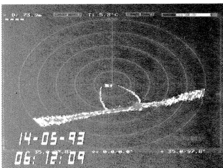
Figur 20. Sonar bilde av Expotrålen før og i to faser av rørplassering. Fase 1: Trål normal før krysning, Fase 2: Trål deformert. Rørledning vises i venstre bildekant, Fase 3: Trålen passerer rørledningen. Rørledningen under babord vinge. [Sonar display of the Expo trawl before and during two phases of crossing the pipeline. Phase 1: the trawl in a normal position before crossing the pipeline; phase 2: the trawl is distorted; phase 3: the trawl is crossing the pipeline with its port side wing].
