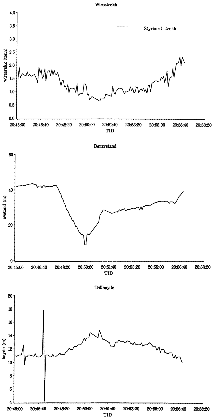
Figur 22. Strekk og geometri av reke-trålen med 25° krysningsvinkel der tråldøren ligger med baksiden ned i ca. 6 min. etter rørpassering. (MS 45, 1. krysning) [ Tension and geometry of the shrimp trawl at a 25° crossing angle, where the trawl door is lying backside down for about 6 minutes after having crossed the pipeline (trawl station no. MS 45, first crossing) ].
