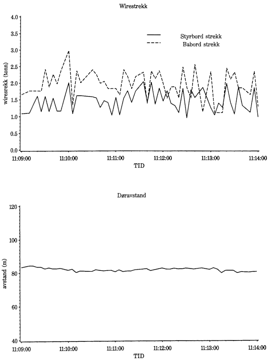
Figur 18. Strekk og geometri av Expo 1200 m/sabb med 40^\circ krysningvinkel (MS 32, 1. krysning) [ Tension and geometry of the the Expo trawl, 1200 meshes with gear, at a 40^\circ crossing angle (trawl station no. MS 31, first crossing) ].
