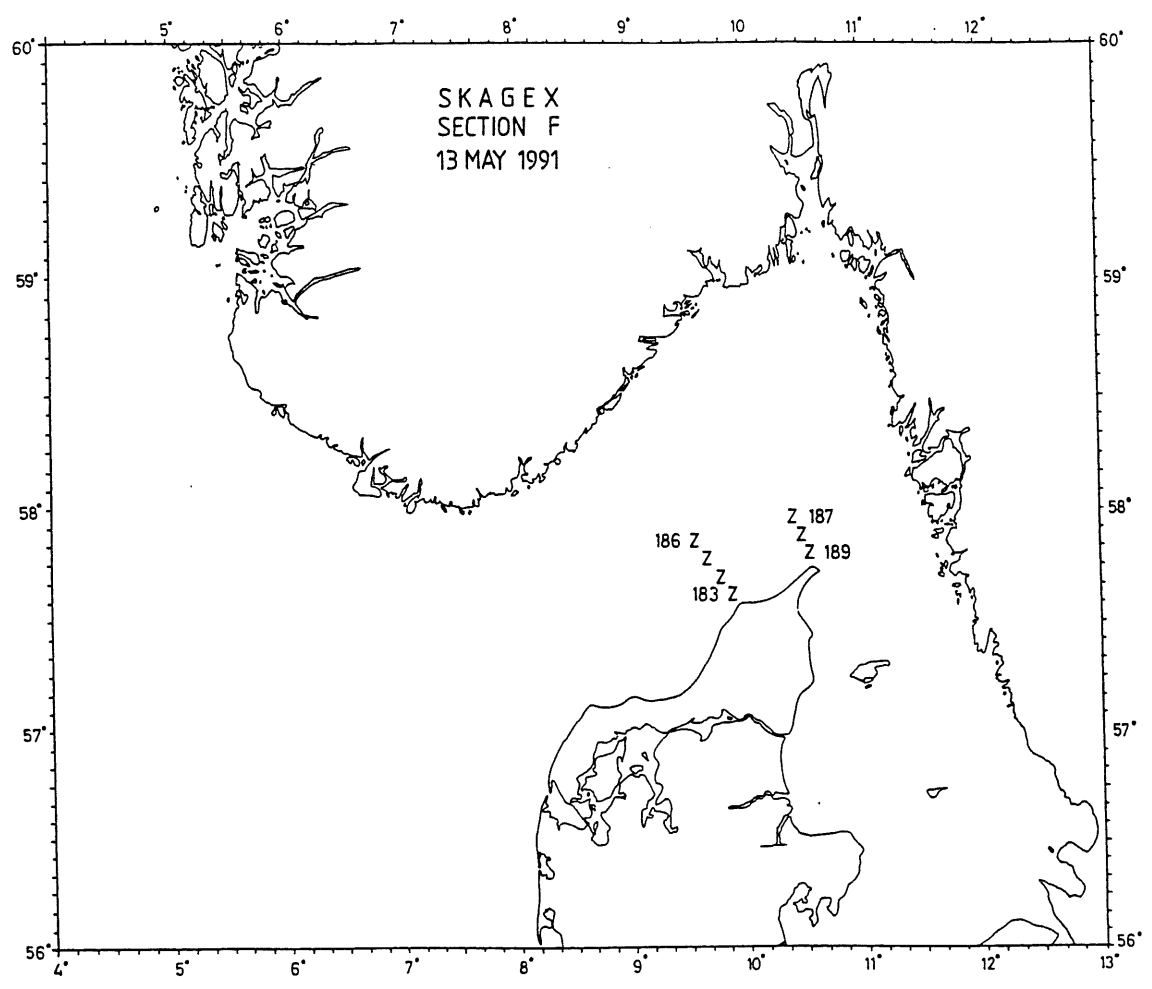
Fig. 1. Stasjonsnettet for G.M. Dannevig 12. - 19. mai 1991 under SKAGEX IV.
