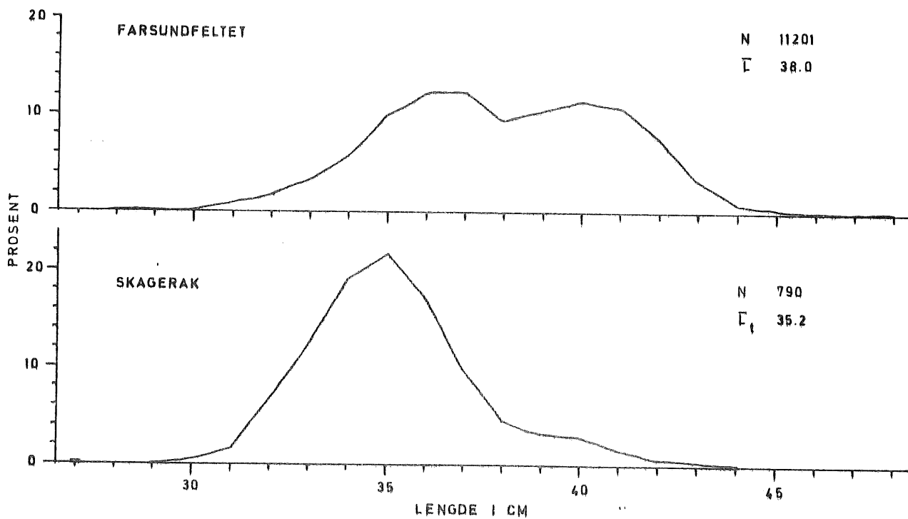
Figur 2. Lengdefordeling av merket makrell fra Farsundfeltet og Skagerak
