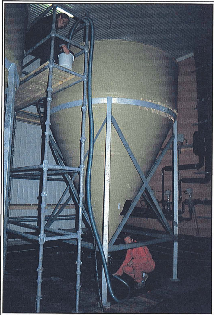
En 15 m 3 inkubator for kveitelarver.
