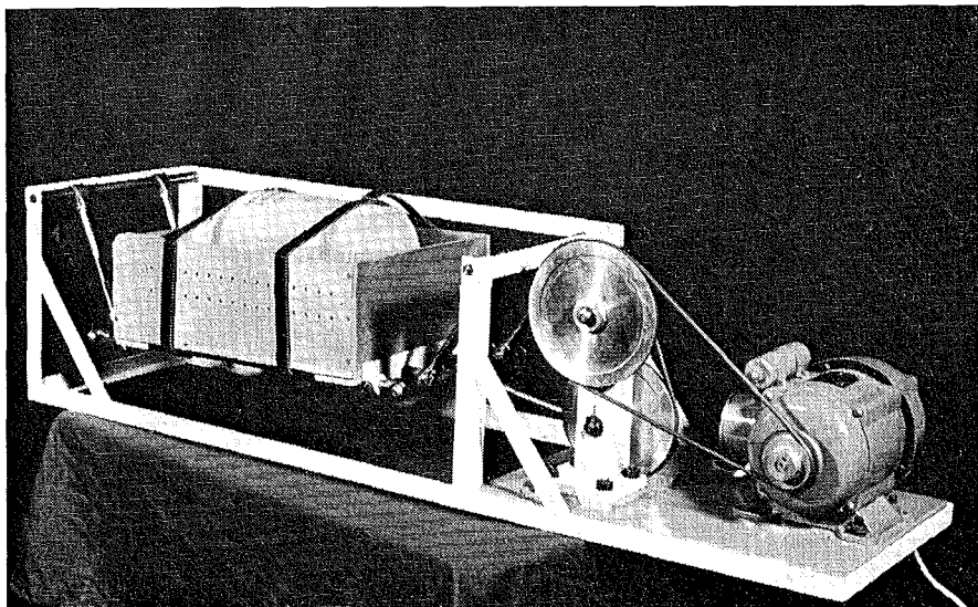
Rystemaskin etter «vugge»prinsippet. Kapasitet 10—15 liter flasker (se forord).
