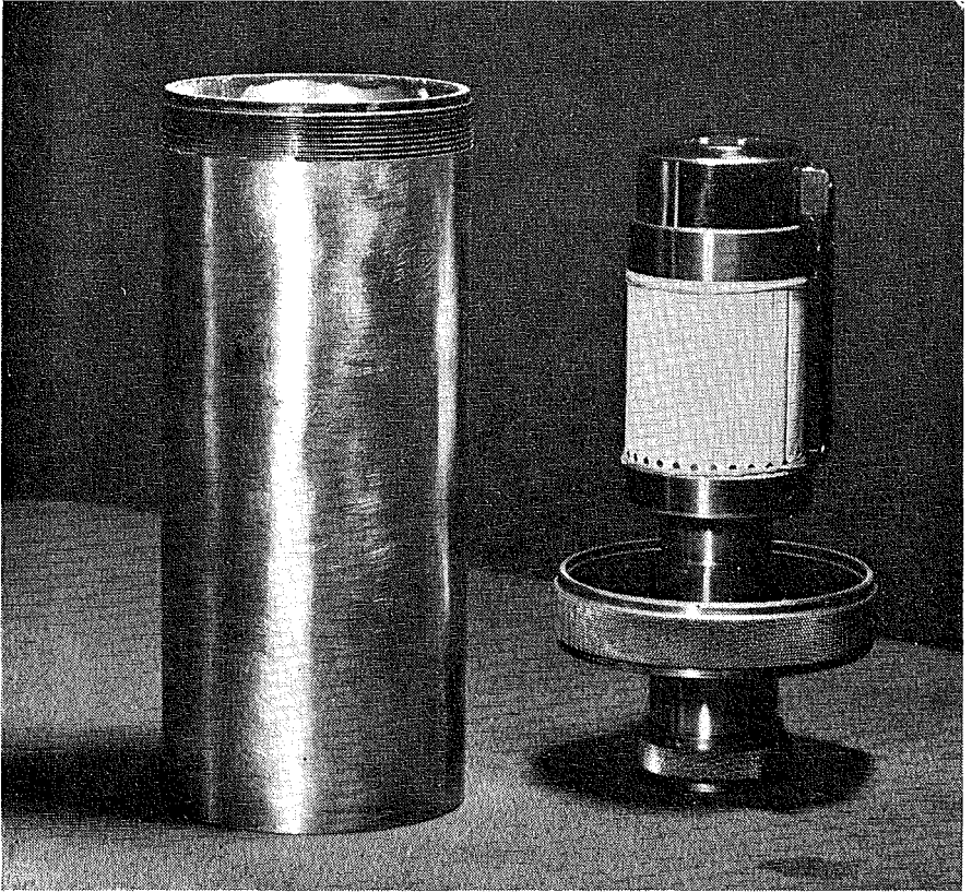
Hesters bathykymograf til måling av synkehastighet og operasjonsdybde for snurpenoter (se forord).
