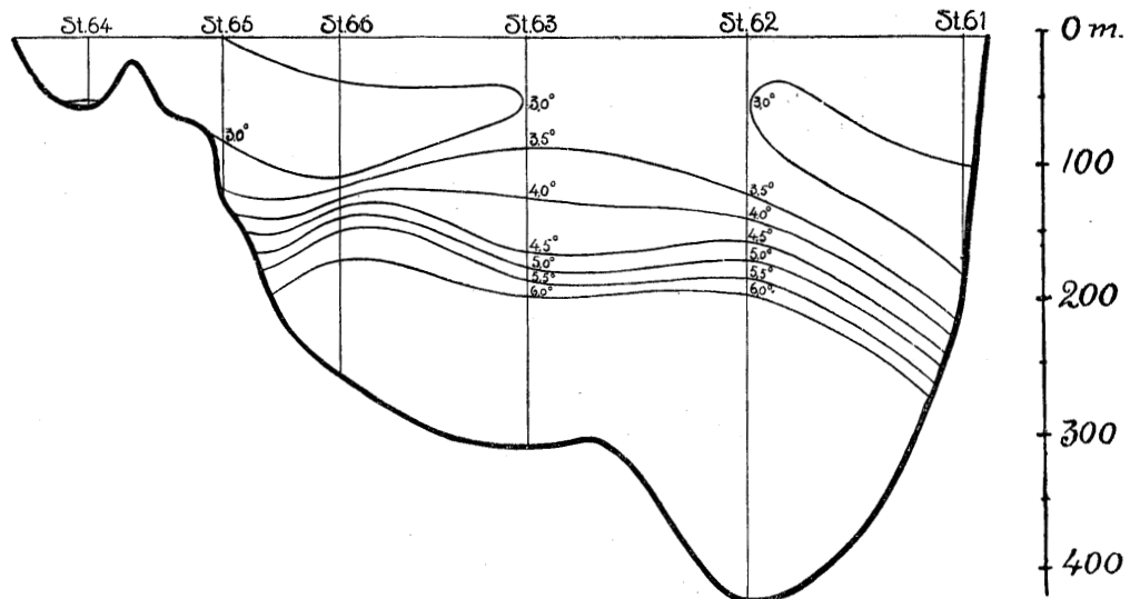
Fig. 129. Gröttö section (cf. Fig. 127). 3° = 3° C.
