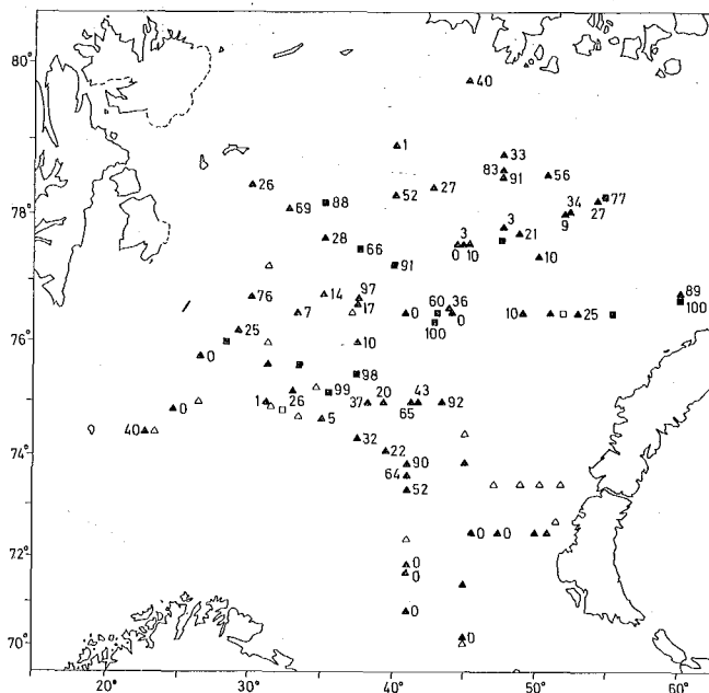
Fig. 9. Ekkomengde av polartorsk i 0—300 m 12.—29. september. [Echo abundance of Polar cod in 0—300 m 12—29 September]
