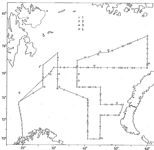
Fig. 1. Kurser og stasjoner 23. august-9. september 1971. 1) Hydrografisk st. med TSD sonde, 2) hydrografisk st. med vannhenter, 3) pelagisk trålst., 4) bunntålst. [Survey route and grid of stations 23 August-9 September 1971. 1) Hydrographic st. with TSD sonde, 2) hydrographic st. with water bottles, 3) pelagic trawl st., 4) bottom trawl st.]
