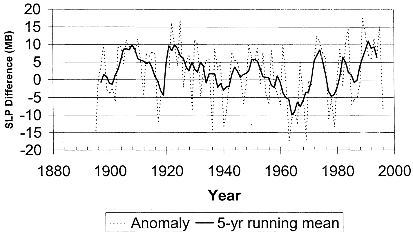
Fig. 4 NAO Index Anomalies
