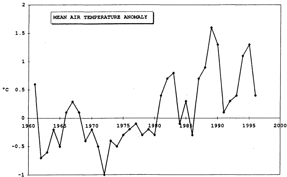
Figure 2. Anomalies in annual mean temperature relative to the 1961-1990 mean. Centro Meteorológico de Santander. Instituto Nacional de Meteorología.
