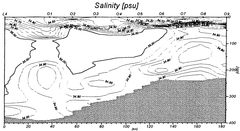
Fig. 3 AREX'95 Confluence Zone
