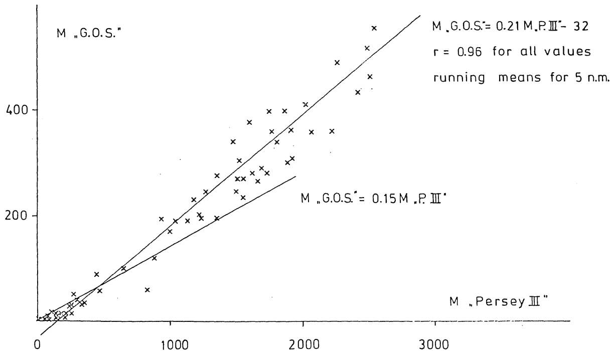
Annex Figure 4. Integrator values „Persey III“ ref. integrator values „G.O.Sars“
